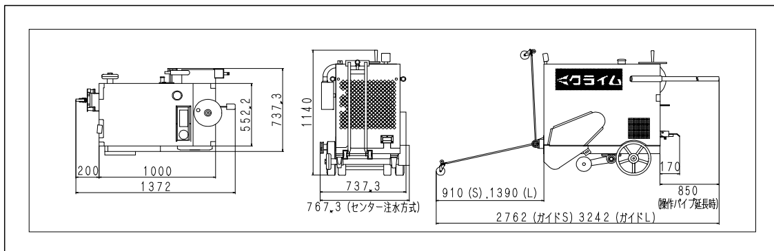
寸法図
