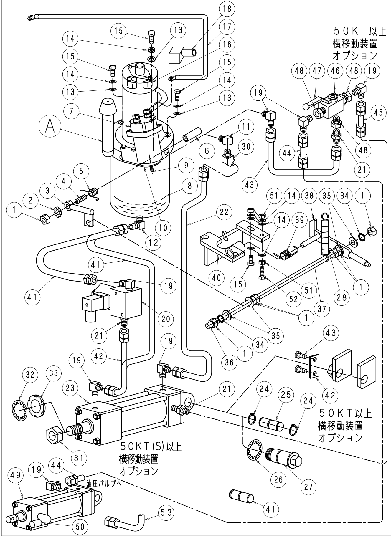
FIG-9 油圧系
