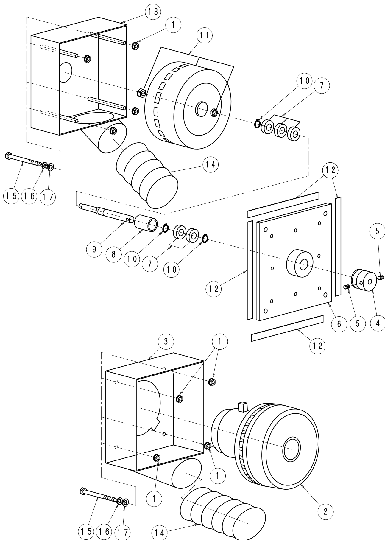
FIG-16バキューム系
