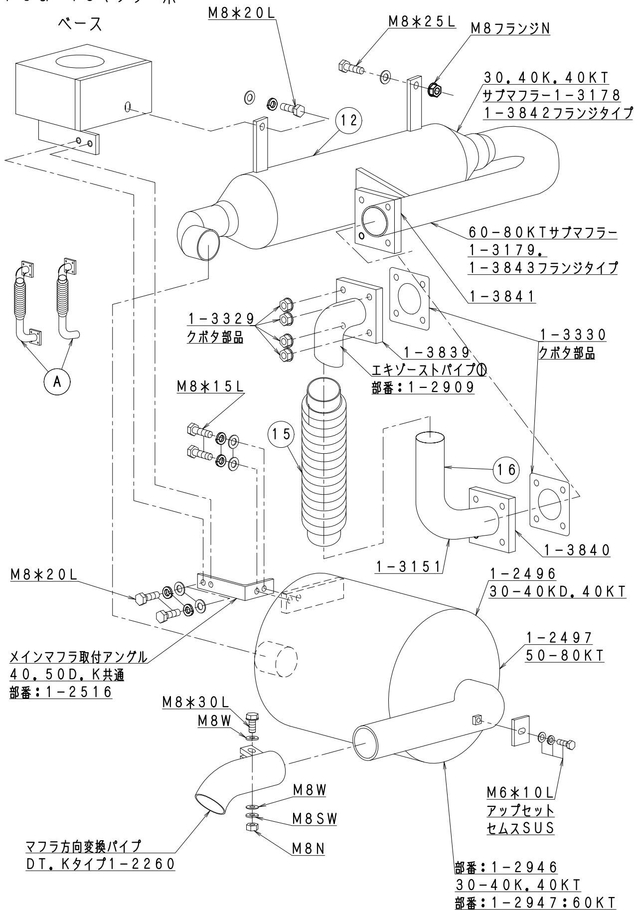
FIG-13マフラー系
