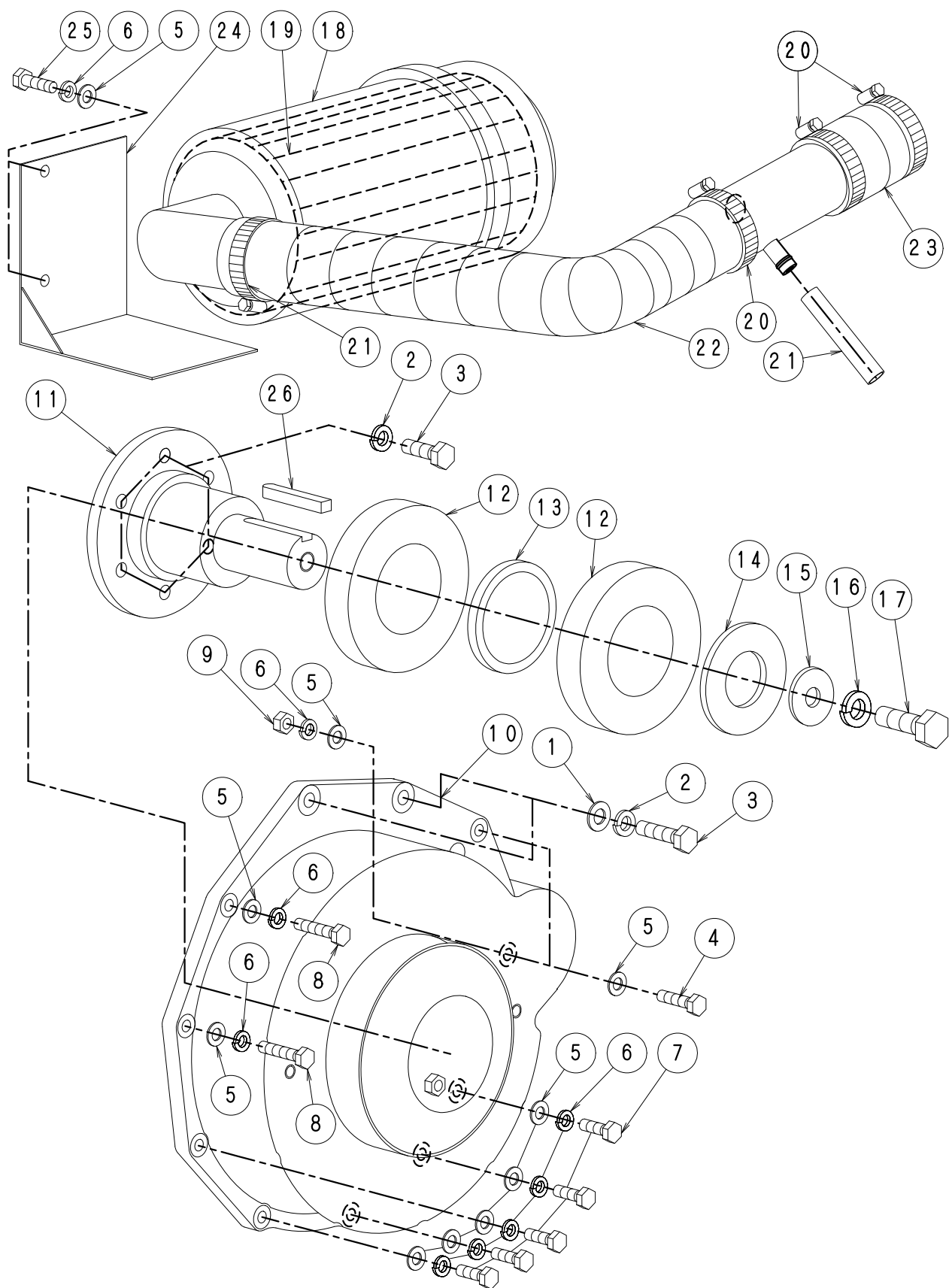
FIG-14-1エンジン系
