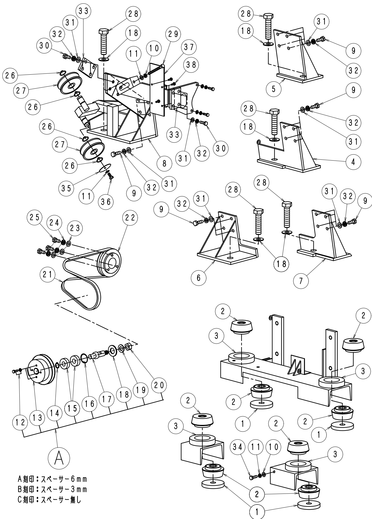
FIG-10 ファンプーリー、マウント系
