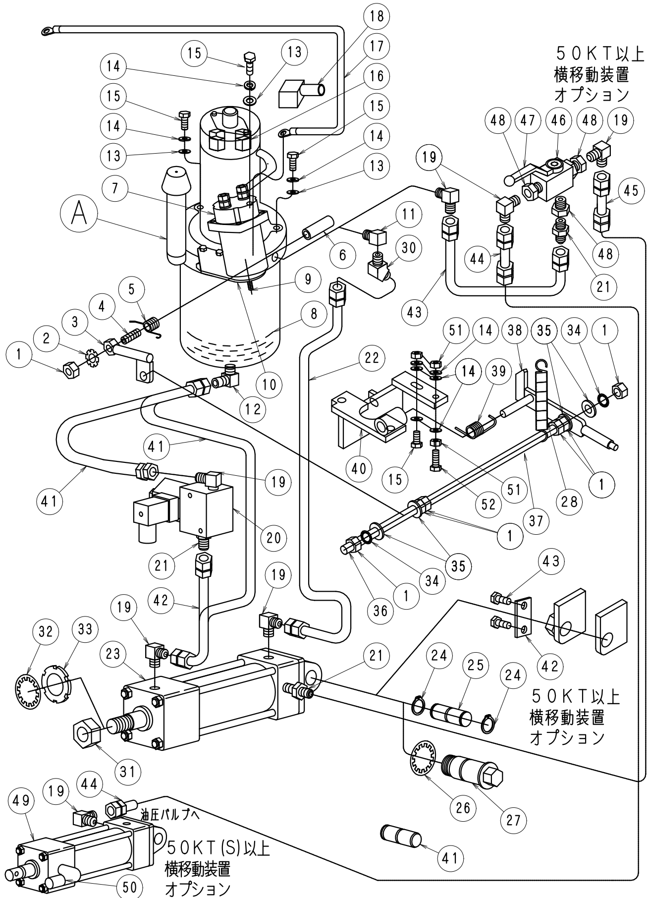
FIG-9 油圧系
