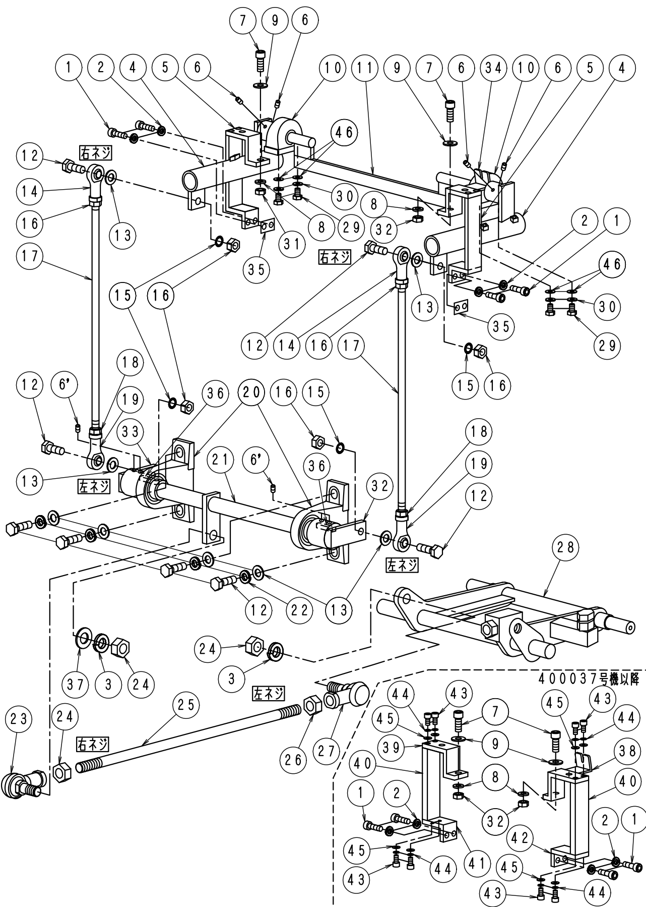
FIG-12 可変操作系
