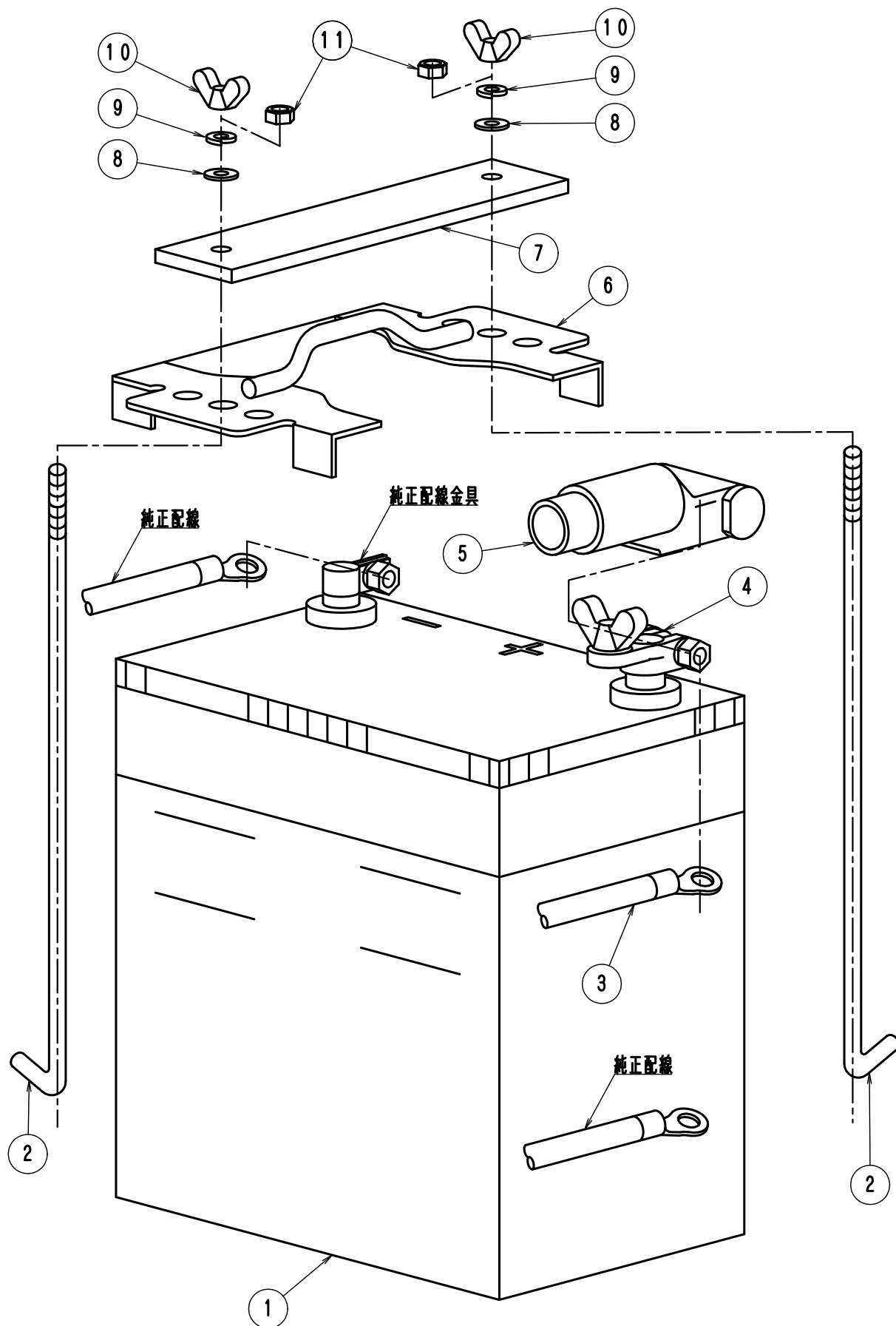
FIG-7バッテリー系
