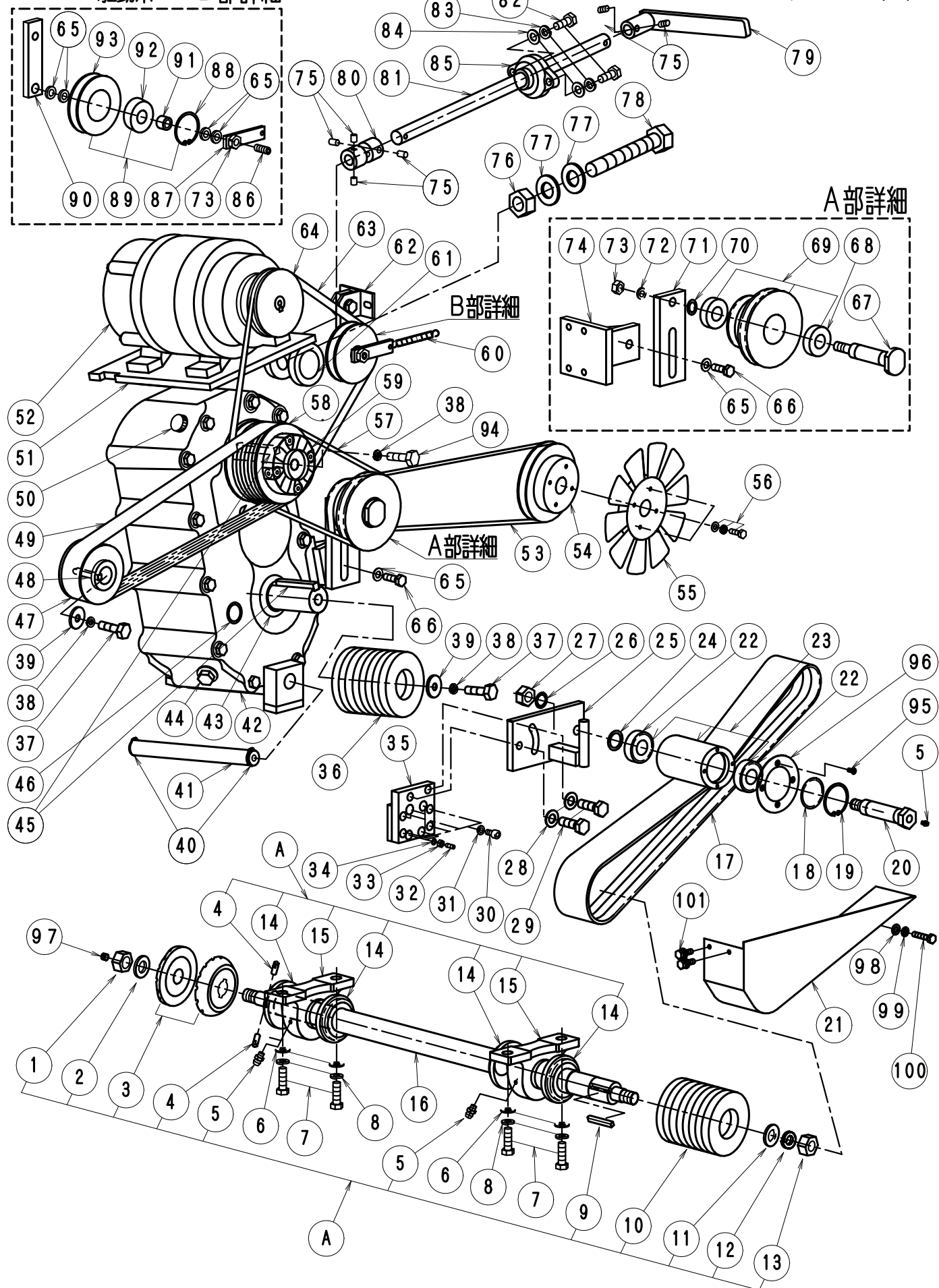
FIG-1 駆動系 B部詳細
