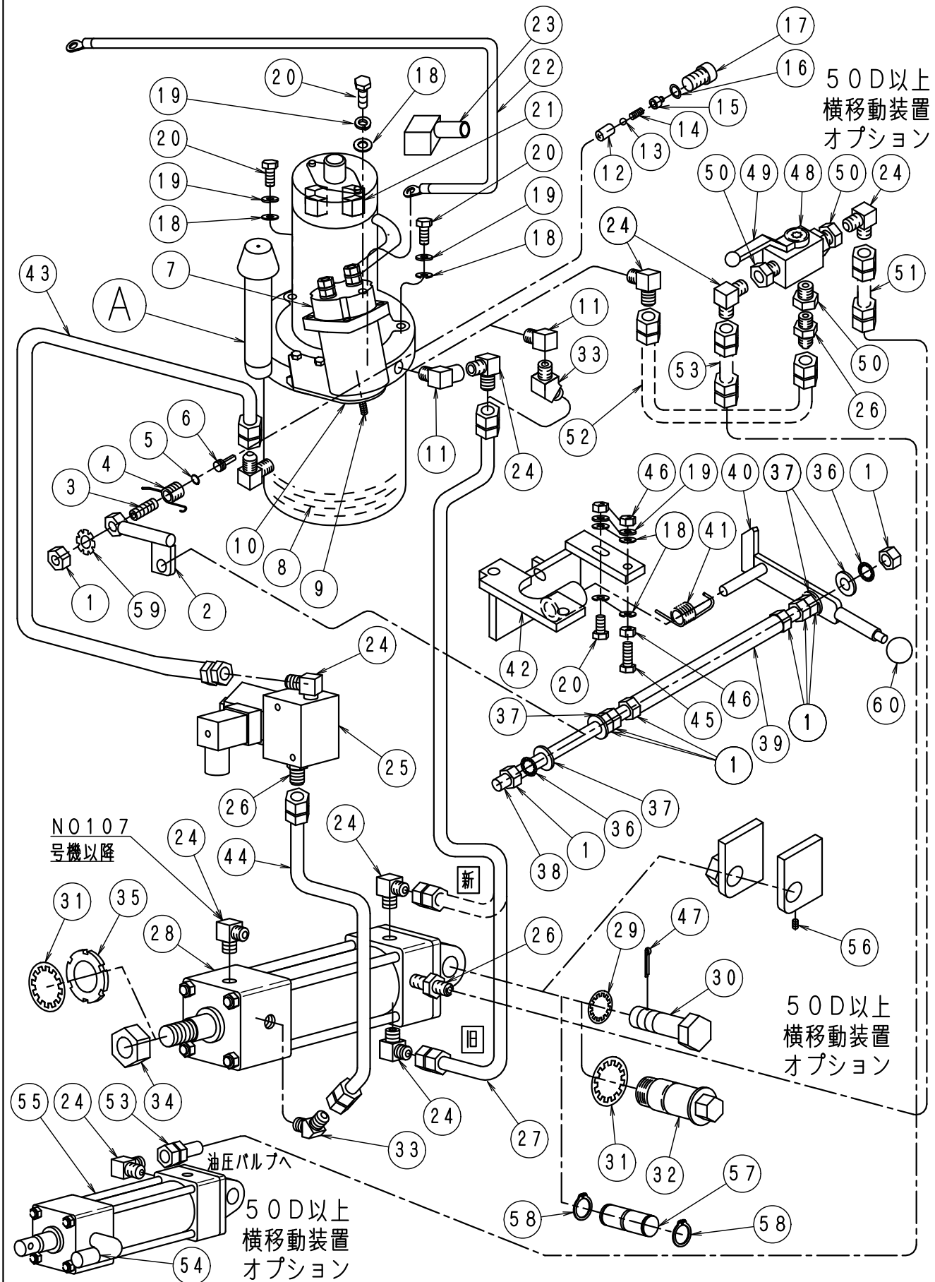
FIG-9 油圧系
