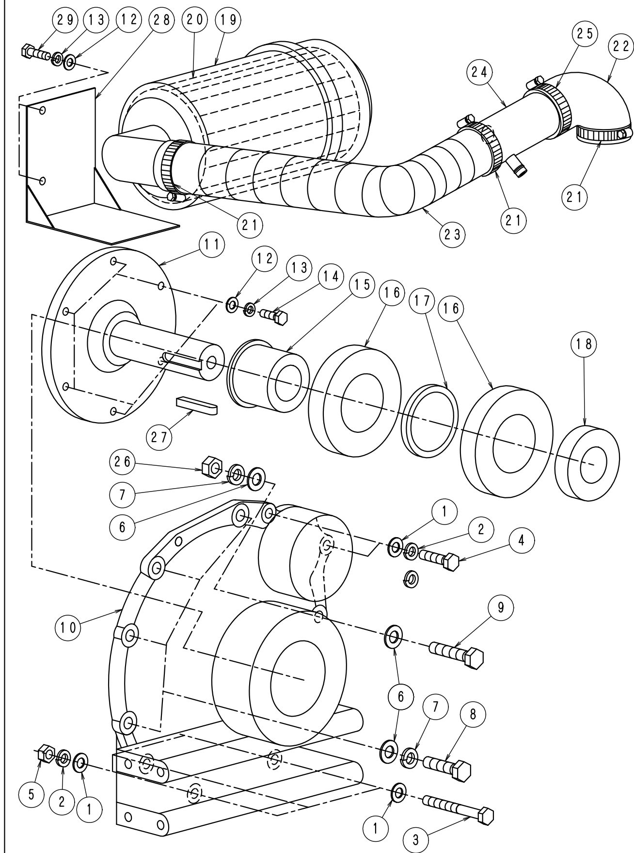
FIG-14エンジン系
