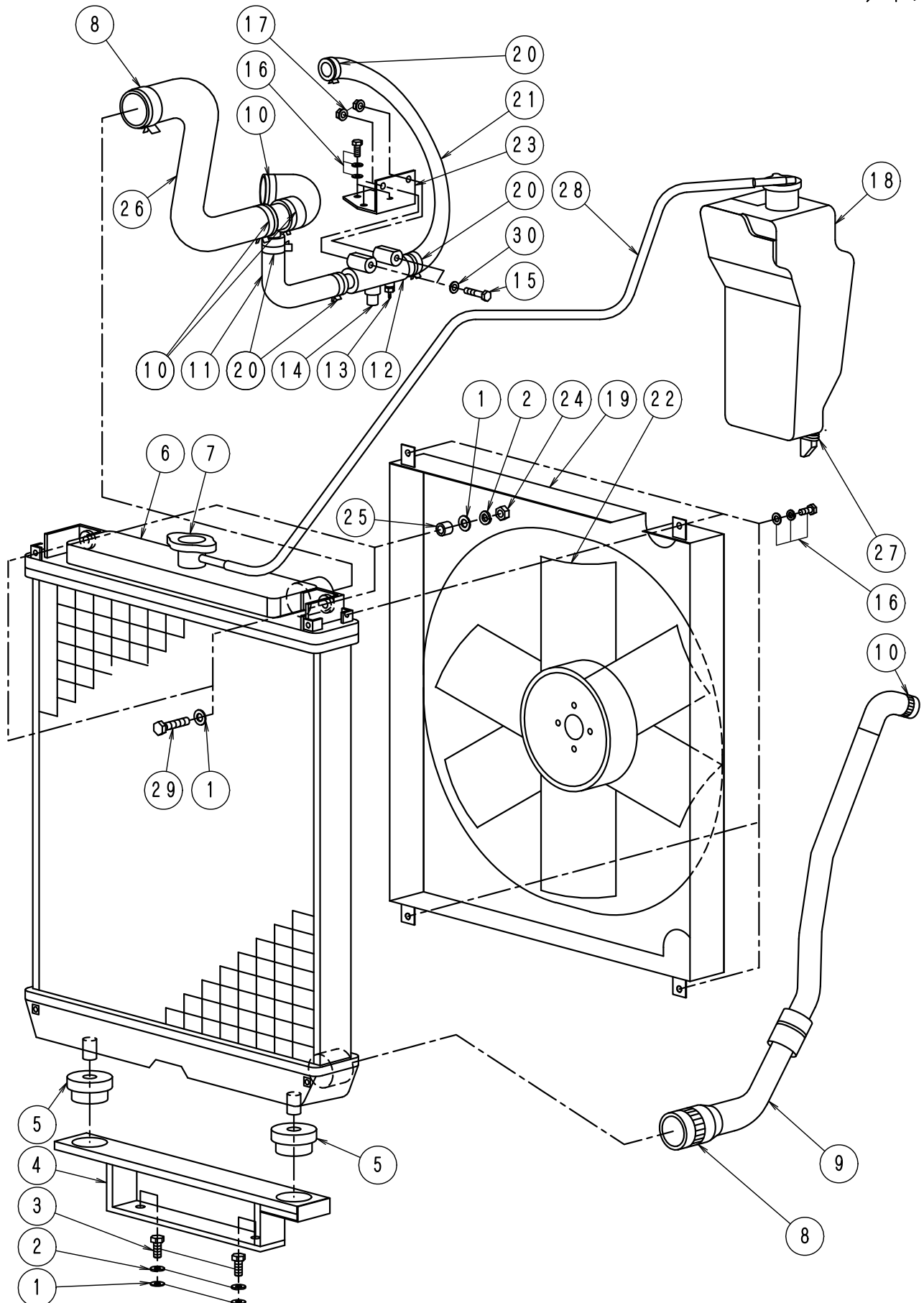
FIG-15 冷却系
