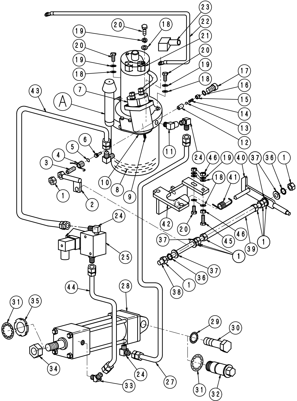
FIG-9油圧系
